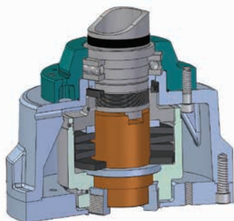
Компенсатор осевого усилия от Rotork.
